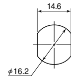
取付穴参考寸法 Mounting Hole
